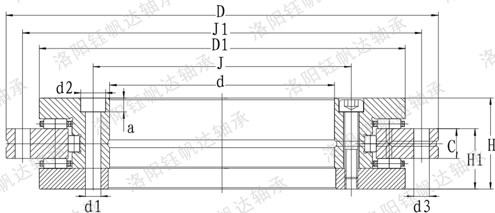
ZKLDF系列转台轴承
